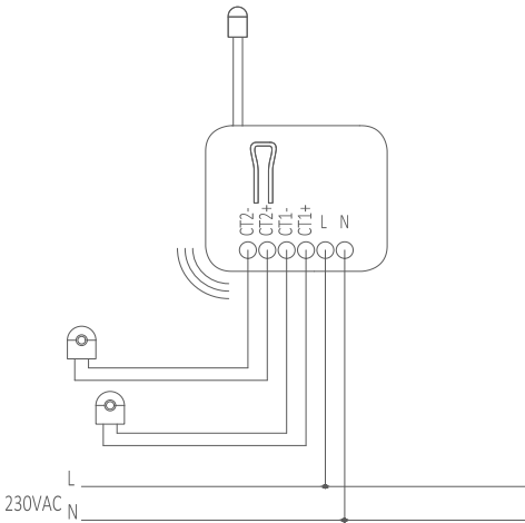
Diagramas de conexión
